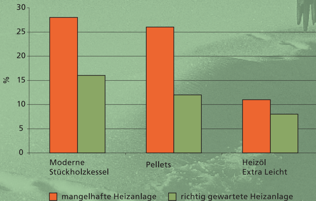
Energieverlust in Abhängigkeit vom Wartungszustand
